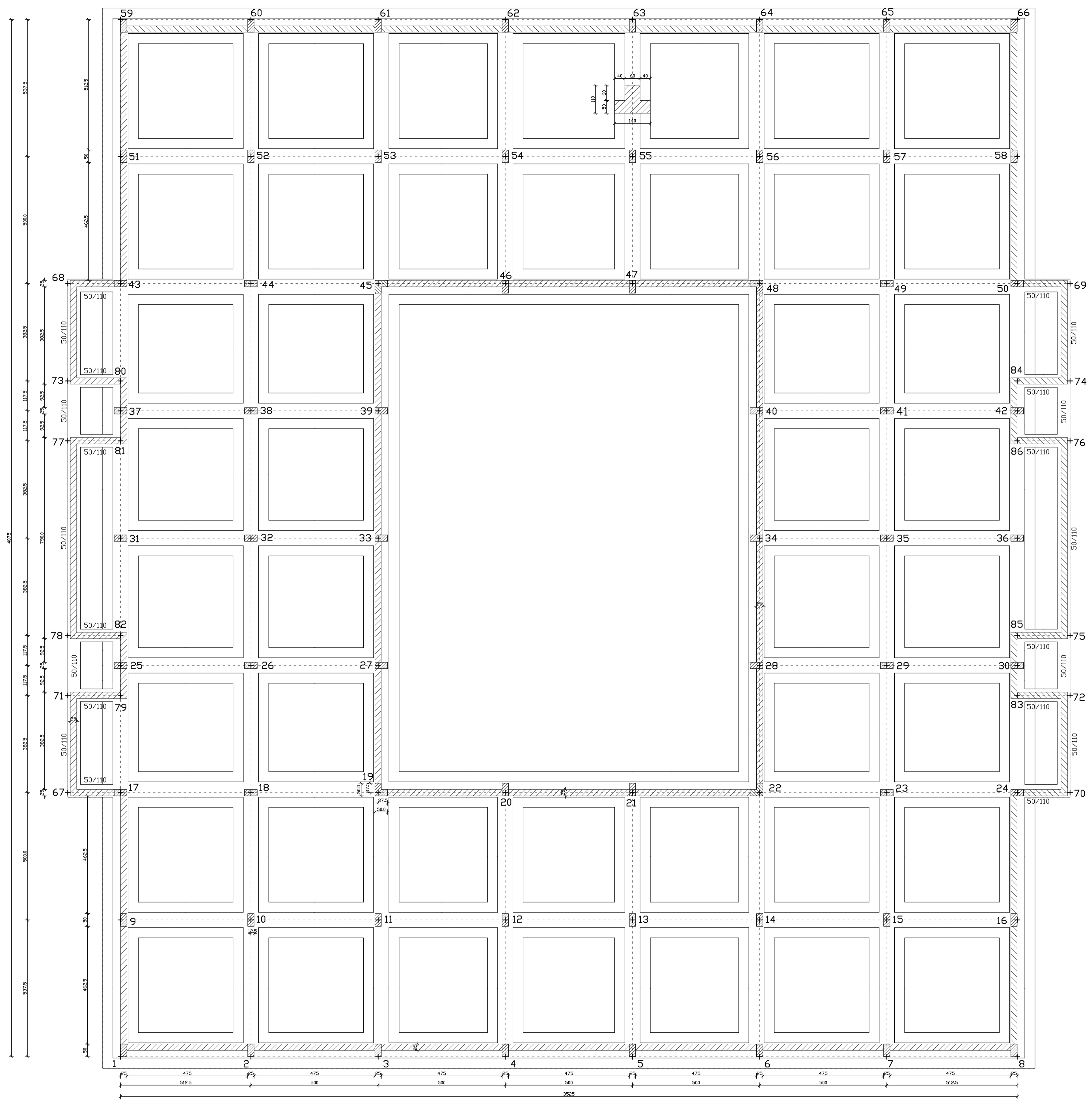
CARPENTERIA FONDAZIONI QUOTA m 0.00
